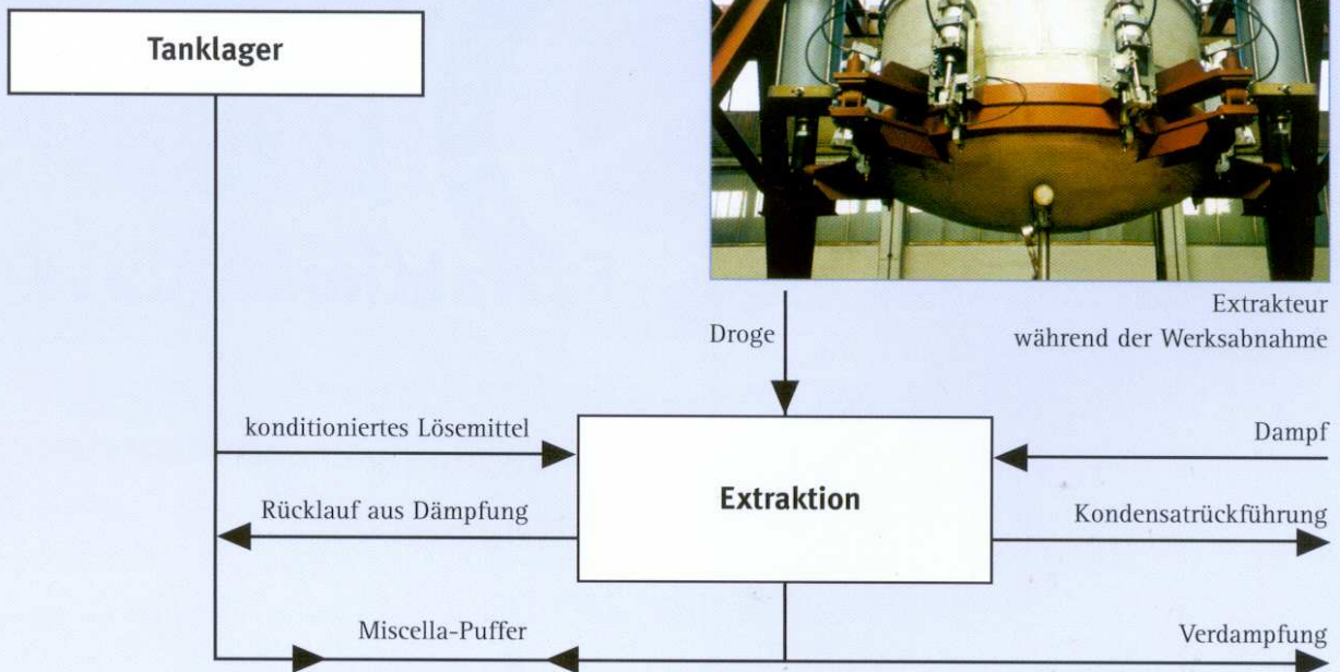
Produktfluss-Diagramm einer Schrader Extraktionsanlage
